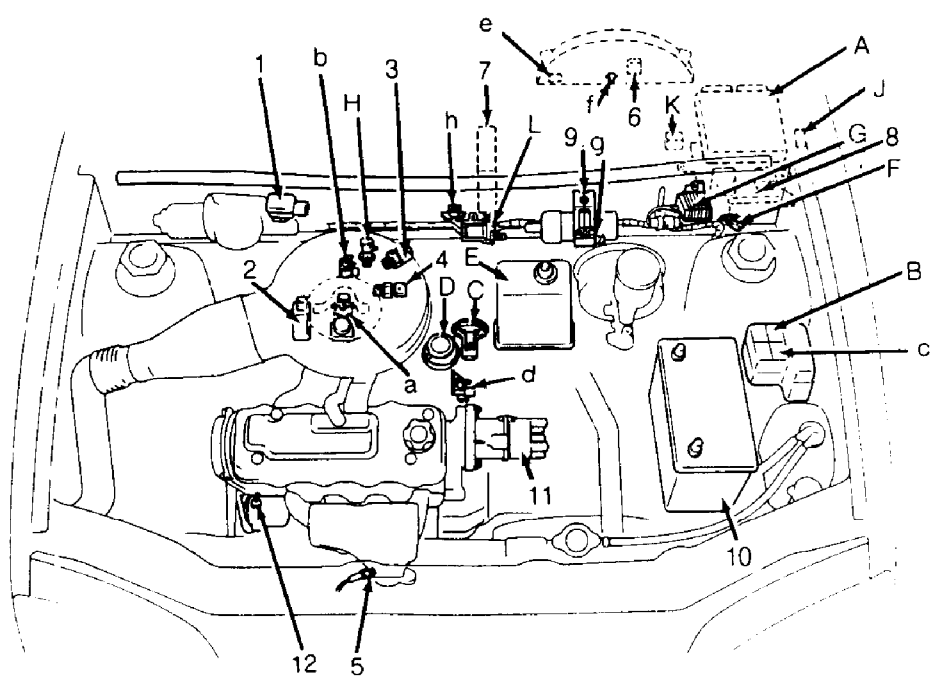
1.3L TBI
