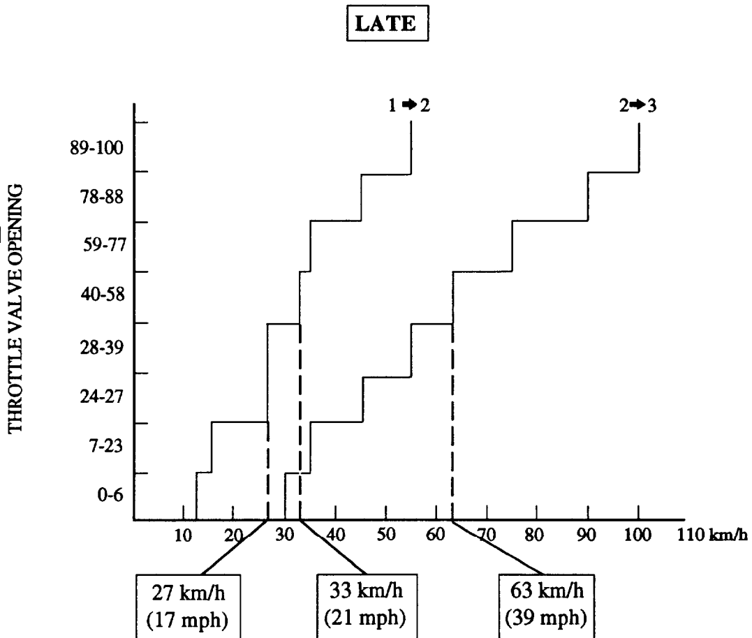
Fig. 3: Revised A/T Shift Diagram
